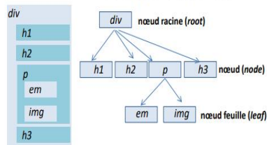
Arbre DOM (Document Object Model)
